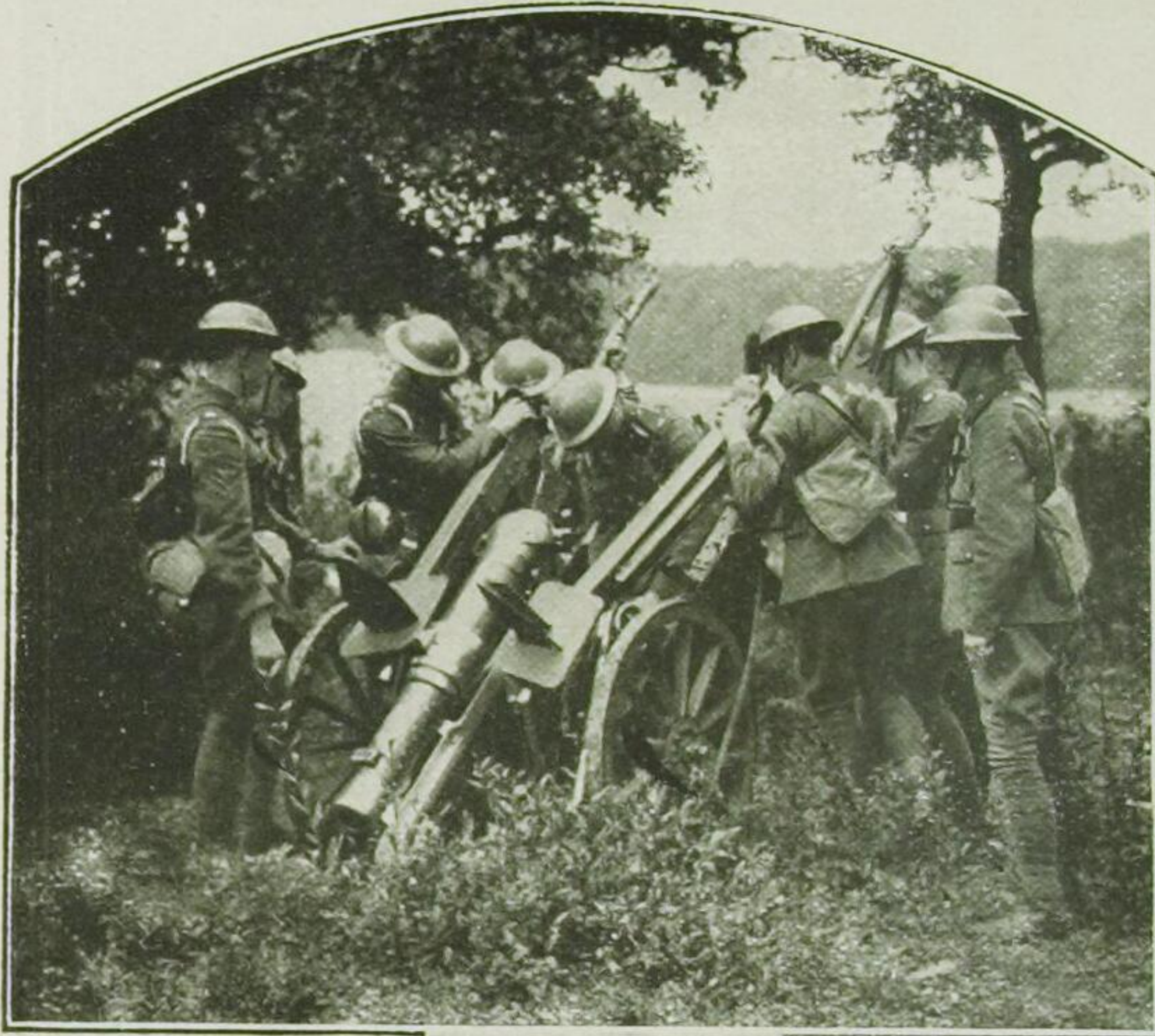
Von den britischen Manövern in Hampshire: Eine leichte Gebirgs- haubitze wird in Stellung gebracht
