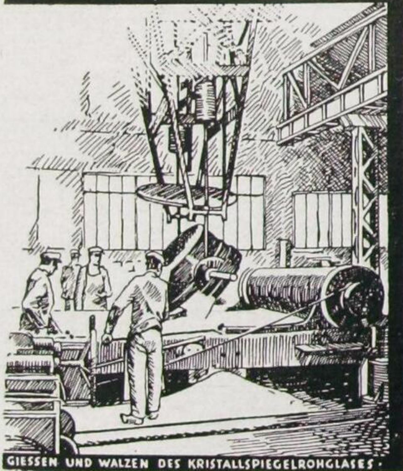
GIESSEN UND WALZEN DES KRISTALLSPIEGELROHGLASES.
