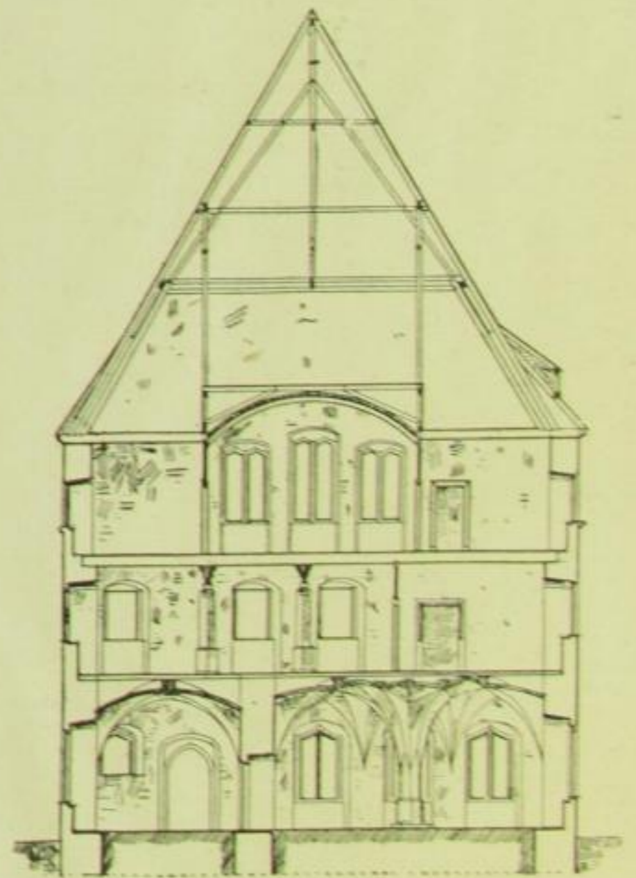
Querschnitt.
