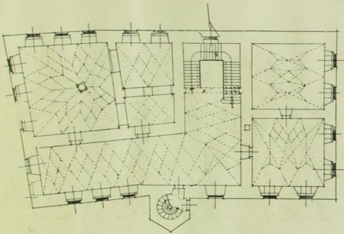
Erdgeschoß.
