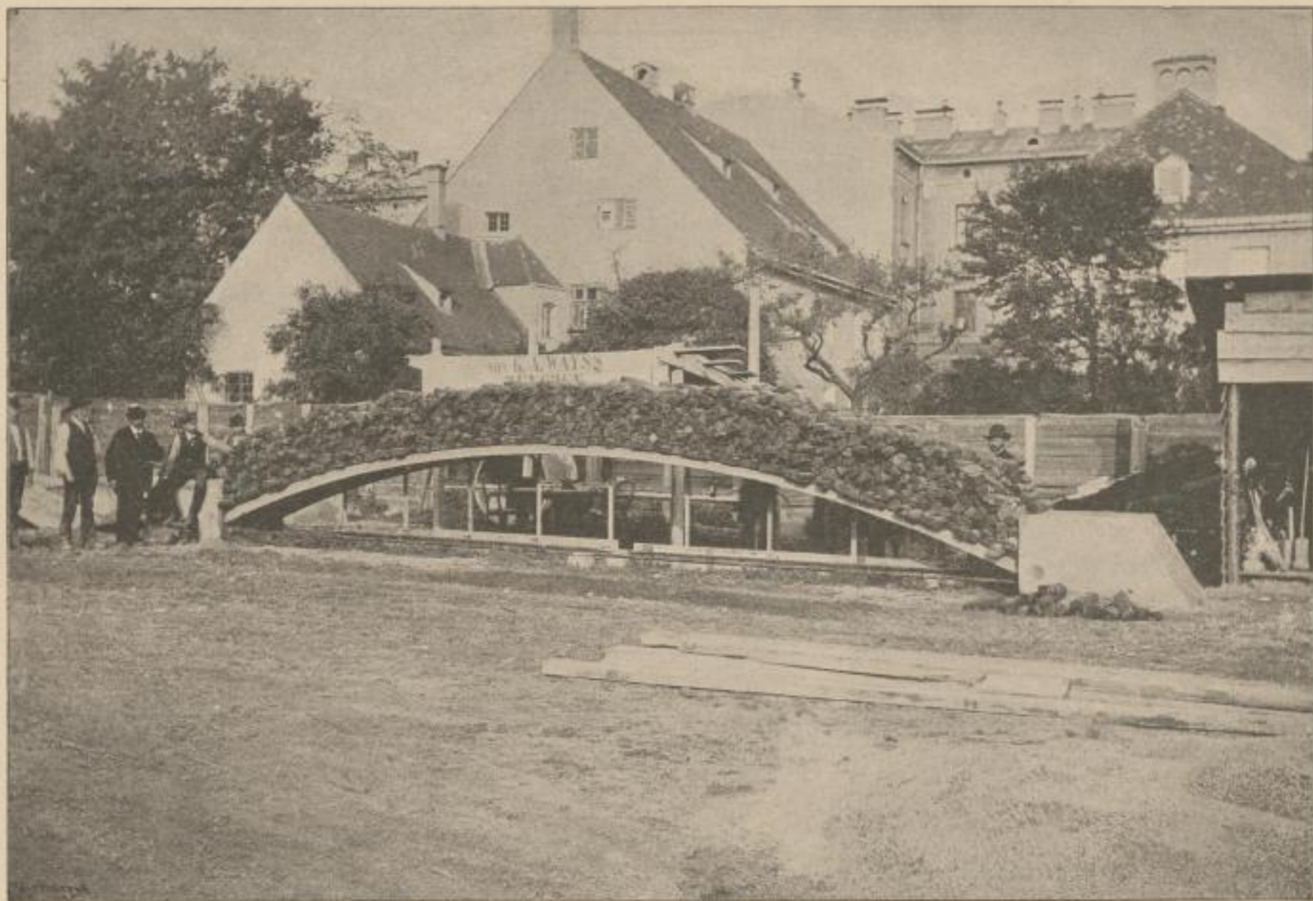
Professor Bauschinger's Belastungsprobe eines Monier-Brückenbogens.
