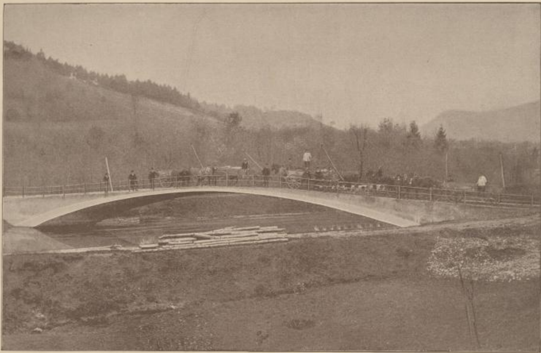
Strassenbrücke nach „System Monier“ bei Wildegg (Schweiz).
