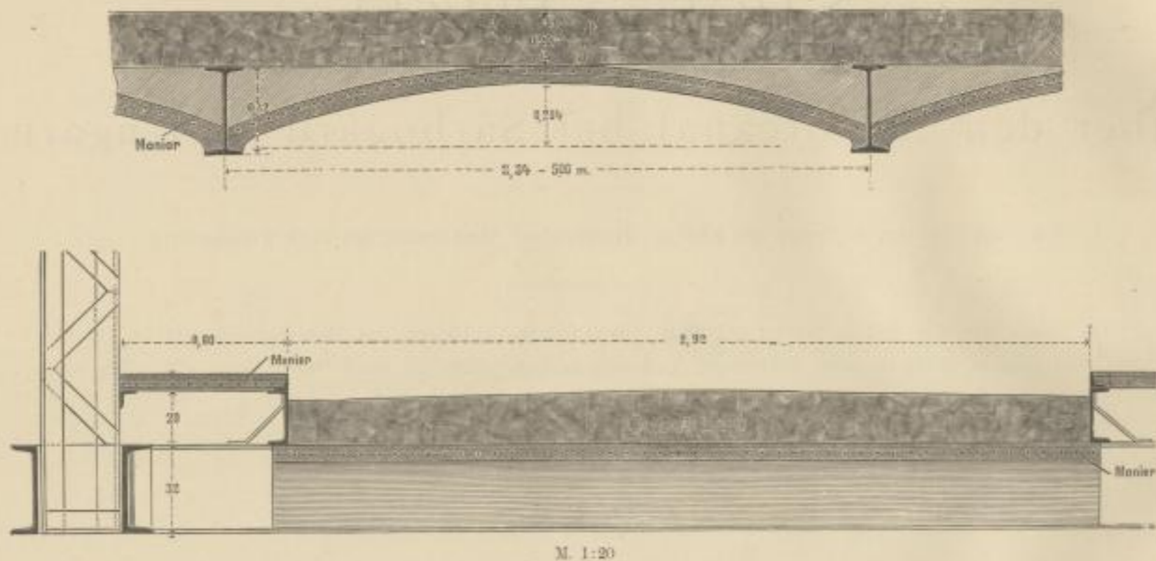
Monier-Abdeckung einer eisernen Brücke.
