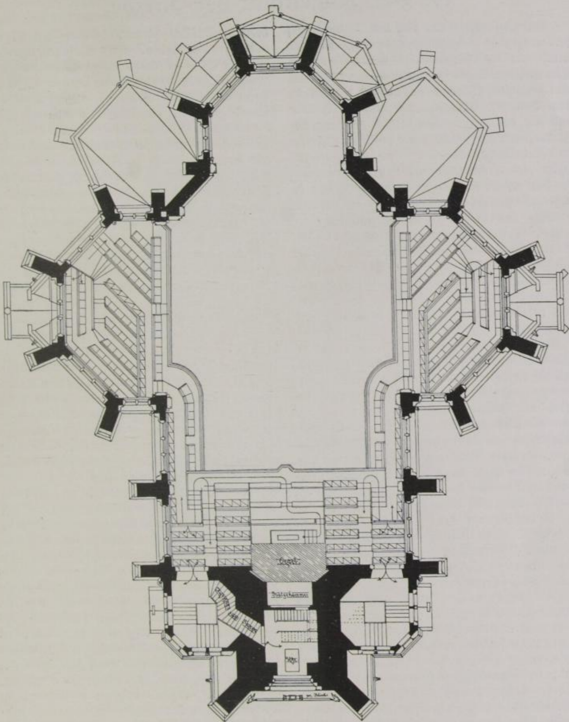
Oberer Grundriß der Kirche. 1 : 250.
