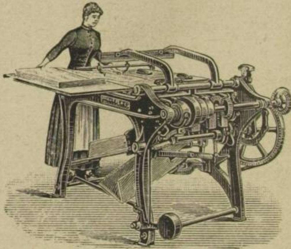
Bogen-Falzmaschine mit Fadenheftung.
