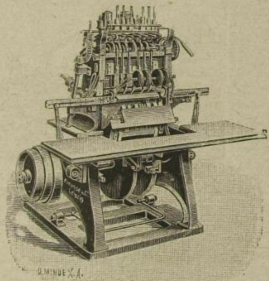
Faden-Buchheftmaschine BB, heftet auf Gaze oder Band.
