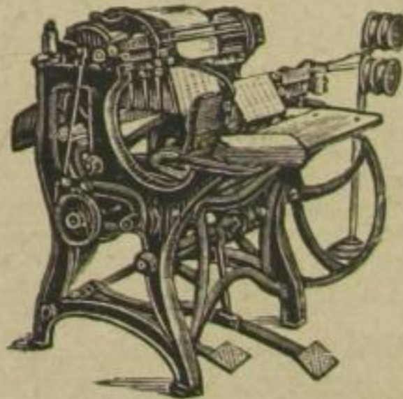
Buch-Drahtheftmaschine „Quarto“
