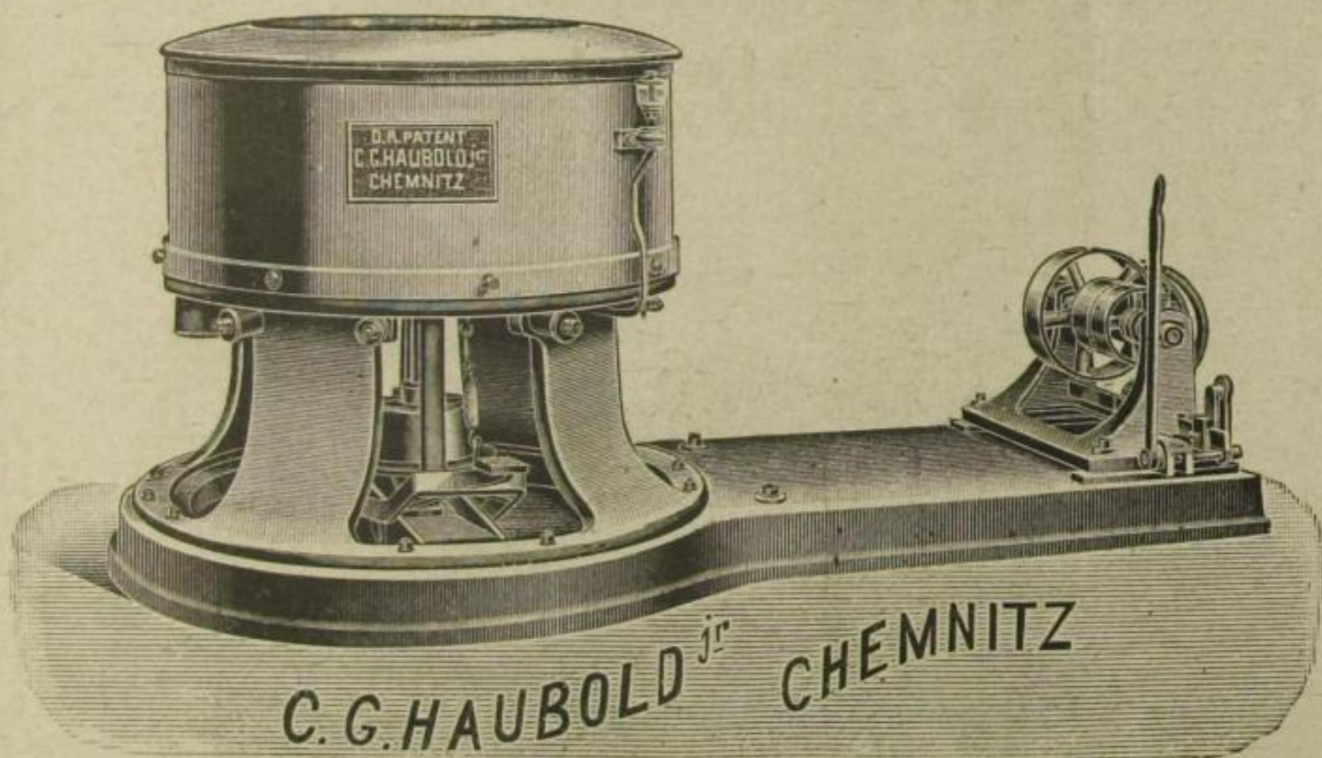
Centrifuge für Transmissionsbetrieb.
