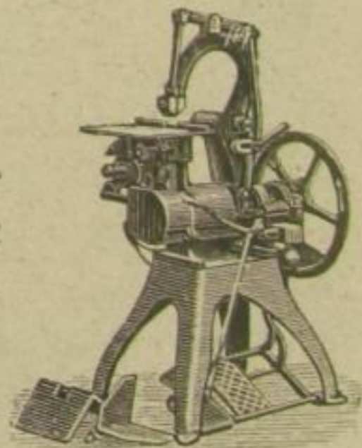
Broschüren-Drahthefmaschinen für Hand-, Fuss- und Kraftbetrieb.
