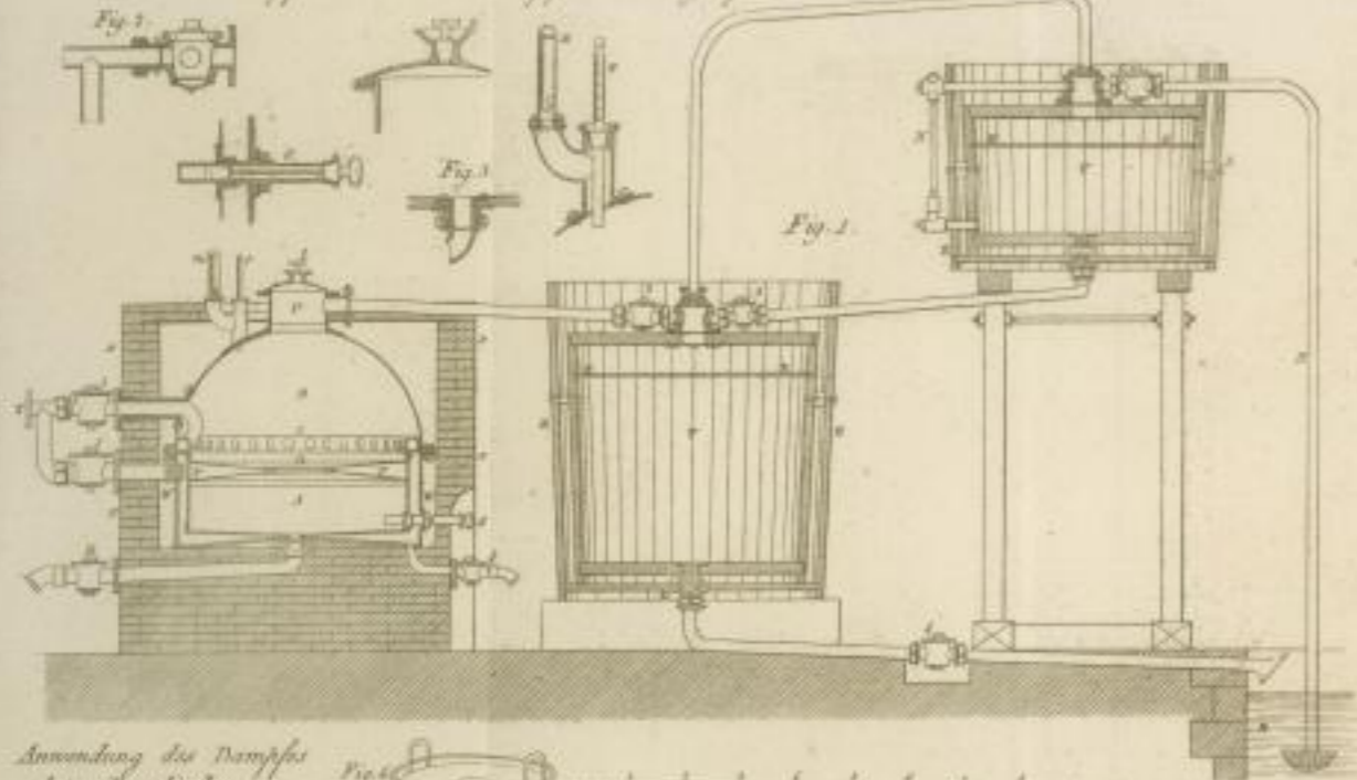
Kochs Apparat zum Verdampfen des Syrups.
