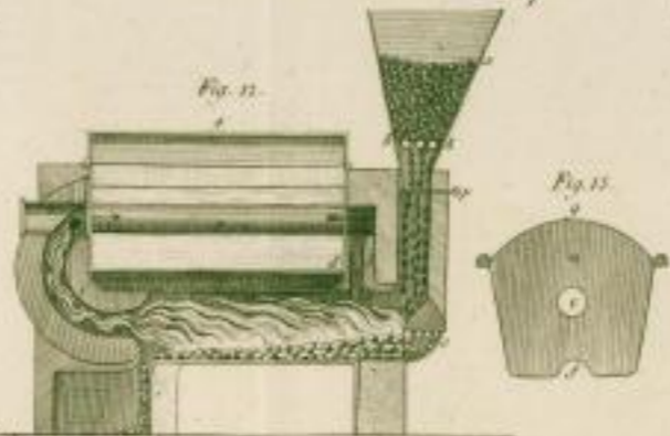
Honell's Patent Ofen zur Erzeugung des Stab - oder Hammersteins.
