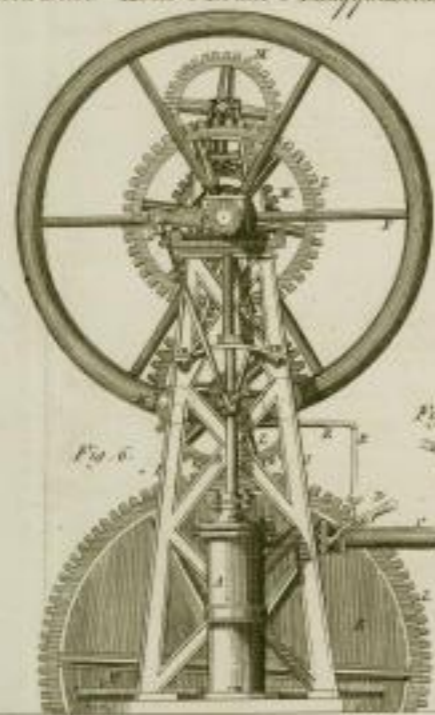
Christie's Hoch-Druck-Dampfmaschine.
