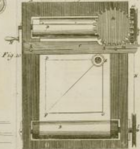
Hudson's verb. Apparat zur Erläuterung der Kältefabriken.
