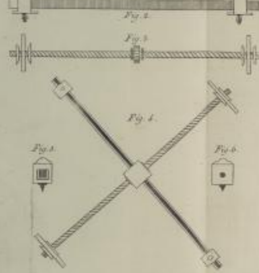
Instrument zum Beschreiben von Spirallinien
