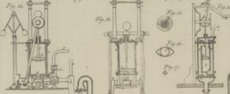
Mallot's Schrauben zum Sprengen der Steine
