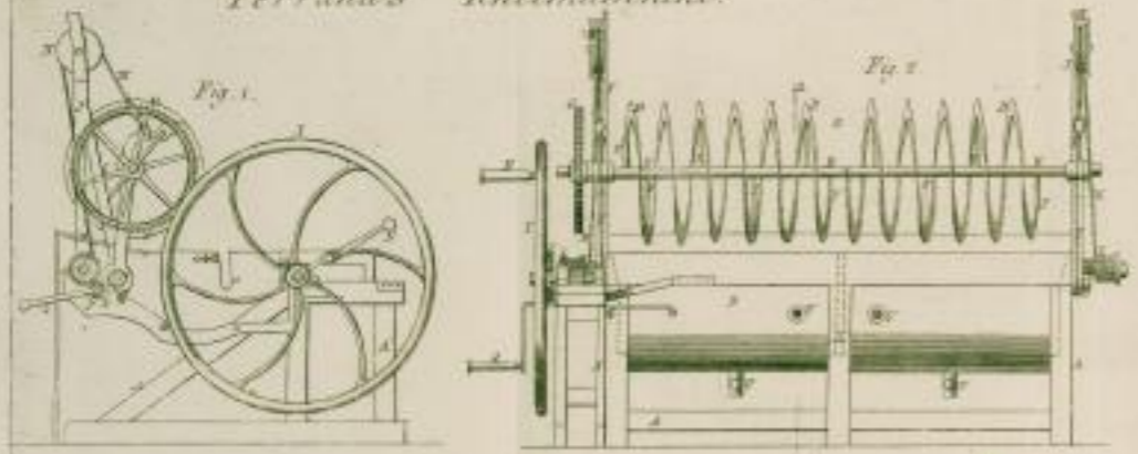
Merrymweather's Apparat.
