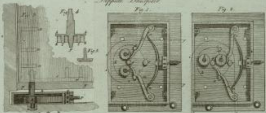
Roberts's Verbindung zur Verbindung der Hauptachsen der Ketten und anderer Schwere
