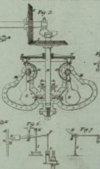
Font und Pumpen Vorrichtung in Kell- und Dampf-Maschinen
