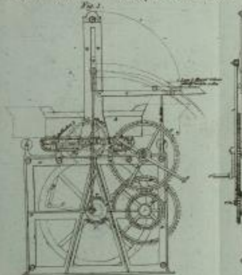
Reine Maschine zum Heben für Wasser zu heben
