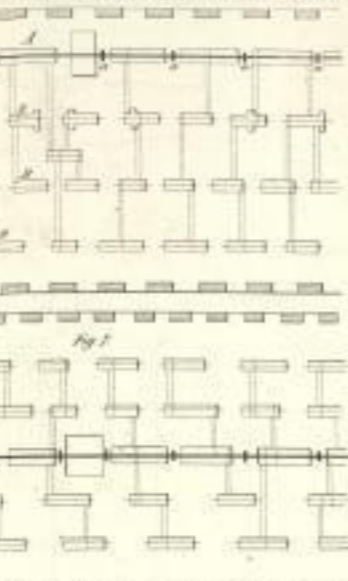
Band oder Petrol der Duane'schen Wellenmaschine
