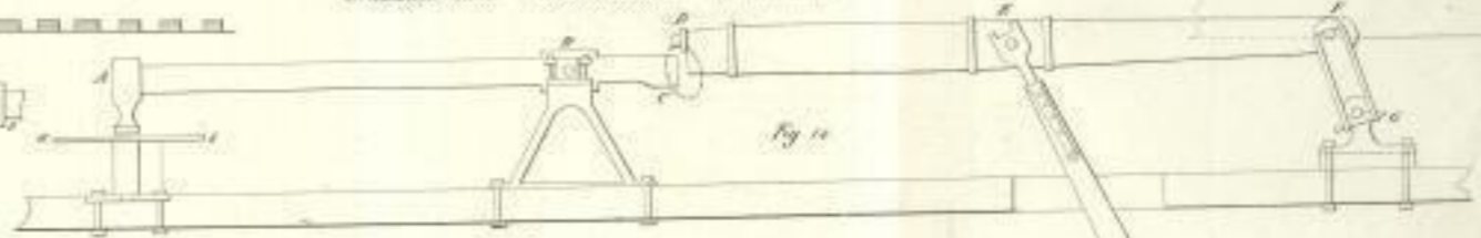
Maschine zum Verarbeiten der Wellen
