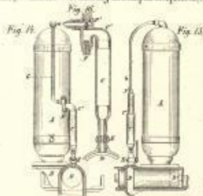
Merryweather's Verbesserung an Dampfdruckspitzen. (Fig. 14-16.)
