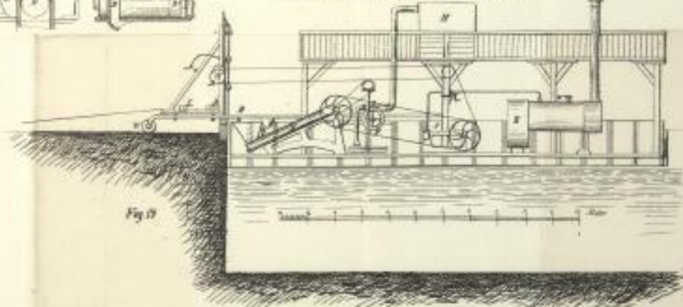
Diebach's System der Torfausbeutung. (Fig. 19.)
