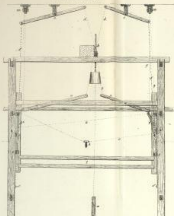
Verbesserung an Differential Rollenzug. (Fig. 8 u. 9.)
