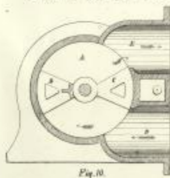
Winder's Dampfzampe. (Fig. 10.)
