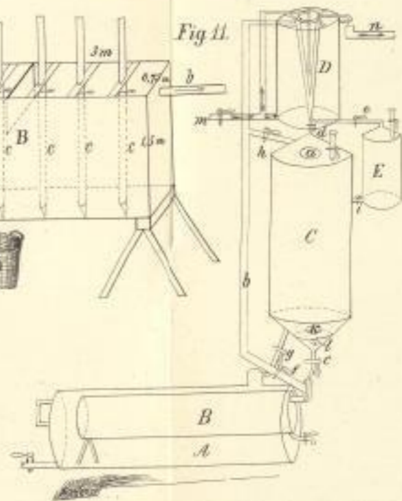
Heuze's Apparate zur Verwerthung der Abgangsweifenwasser. (Fig. 10 u. 11.)
