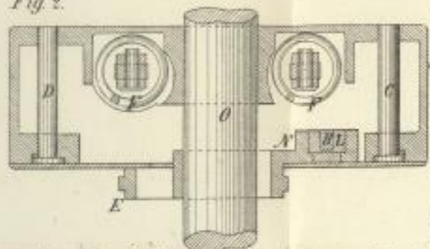
Barometer mit selbstthätigem Registrirapparat. (Fig. 2.)
