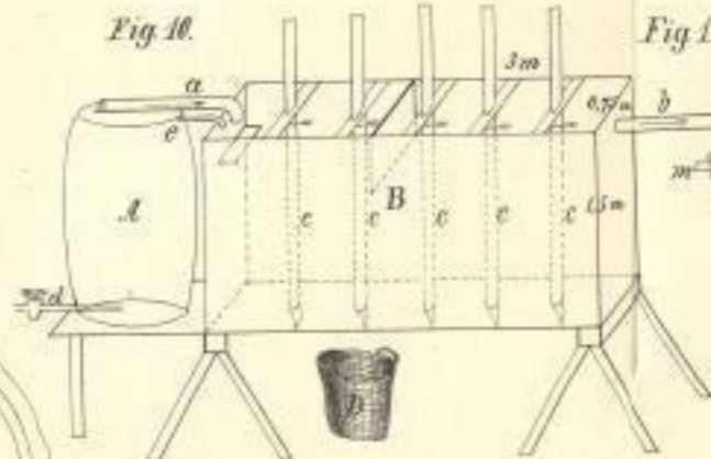
Heuze's Apparate zur Verwerthung der Abgangsweifenwasser. (Fig. 10 u. 11.)
