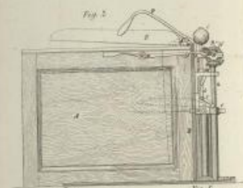
Silvester's Apparat zum Geraderichten von Stahlplatten. Fig. 1, 2, 3, 4, 5, 6, 7, 8, 9, 10
