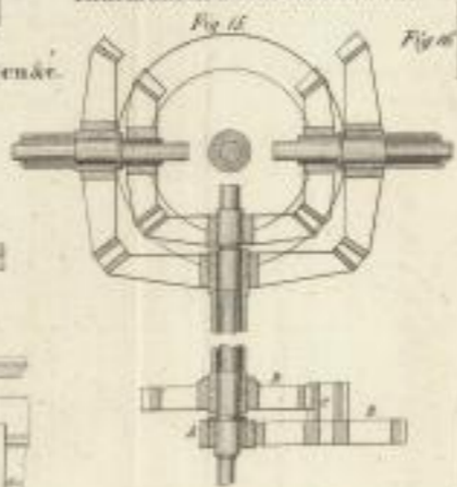
Blaylock's Zeigerwerk für Turmuhren aus vier Zifferblättern. Fig. 15, 16
