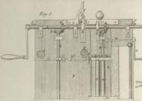
Black's Maschine zum Zusammenfalten des Papiers. Fig. 1
