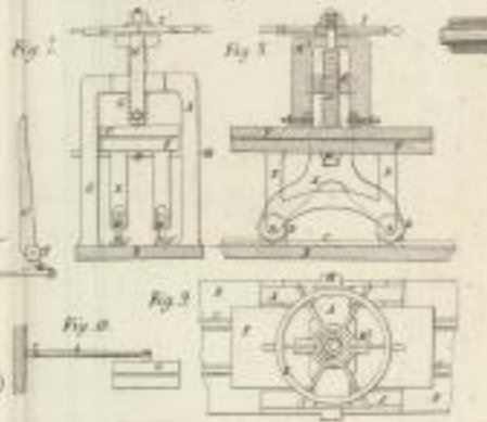
Silvester's Apparat zum Geraderichten von Stahlplatten. Fig. 1, 2, 3, 4, 5, 6, 7, 8, 9, 10
