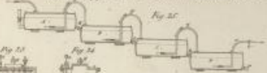
Warmont's Apparat zum Färben von Wollenzügen.
