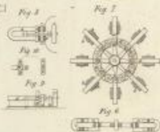
Milward's magnet. elektr. schein Maschinen.
