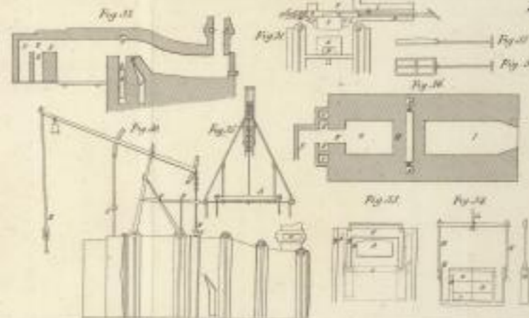
Muntz's Ofen zum Schmelzen von Messing Glockenmetall etc.
