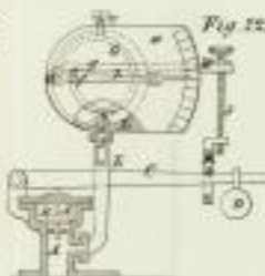
Newton's Druckanzeiger.
