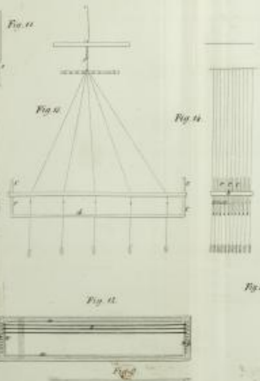
Grothe's Harnisch-Vorrichtung.
