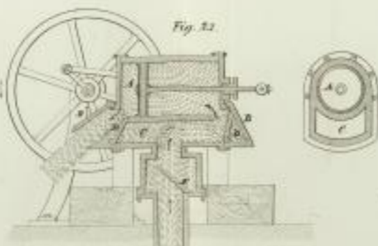
Doppelwirkende Wasserpumpe.
