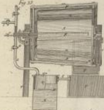
Johnson's Dampf-Reinigungsmaschine für Wäsche.
