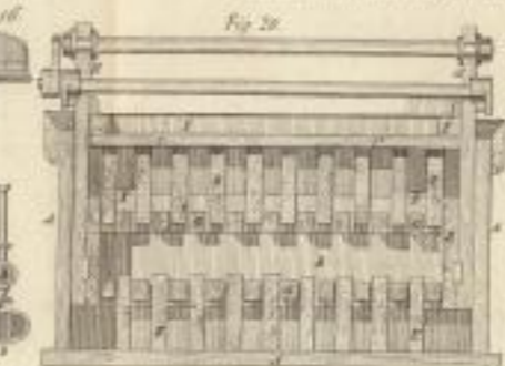
Paterson's Waschmaschine für Zeuge.
