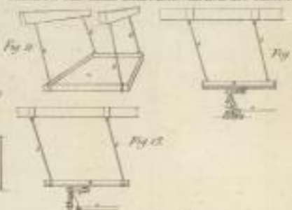
Charré's Maschine zum Mattschleifen des Glases.
