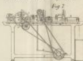
Bary's Maschinen zum Vorbereiten des Flachses für das Verspinnen.
