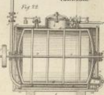
Verschlossene Gefäße zur Stearinsäure-Fabrikation.
