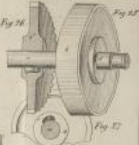
Befestigung von Rollen und Käedern auf Wellen.
