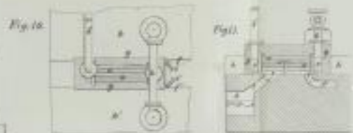
Balbin's Apparat zum Überhitzen des Dampfes.
