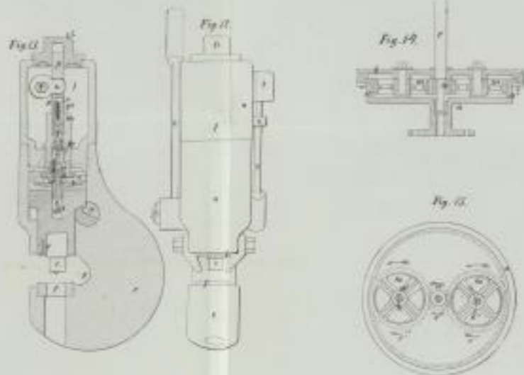
Taylor's Durchstoß mit Anwendung von Wasserdruck.
