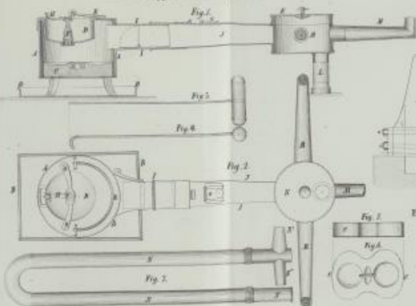
Laxenou's Apparat für Dampfblinder.
