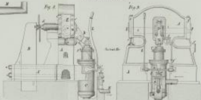
Ecker's Mechanismus zur Bewegung der Rührer und der Flügel bei Kühlschiffen.
