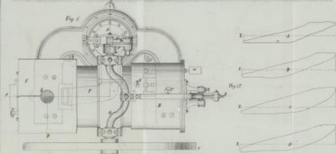
Relative Stellung des Pleuels und Pleuelstange während einer Umdrehung in der Laubert'schen-Schwarzkopfschen Heißluftmaschine.
