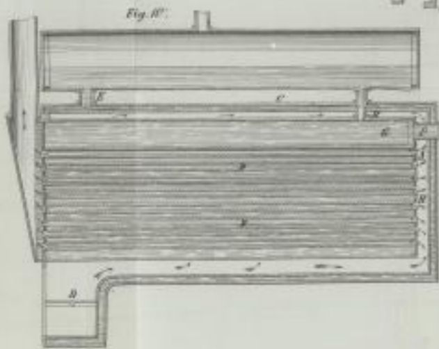
Harris, verbesserter Dampfkessel.
