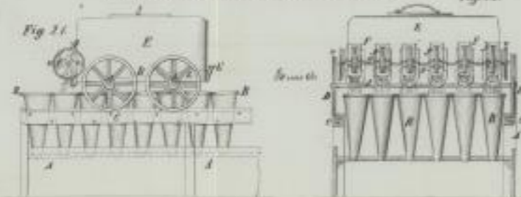
Legals Füllvorrichtung für Zuckerfabriken.
