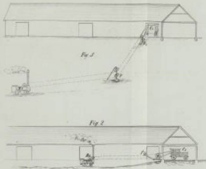
Erkert'sche Drahtseil-Transmission zum Betriebe einer Dreschmaschine.
