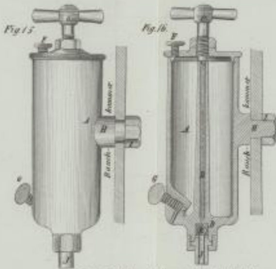
Legals Füllvorrichtung für Zuckerfabriken.
