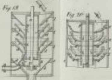
Chester's Maschine zum Trocknen des Getreides.
