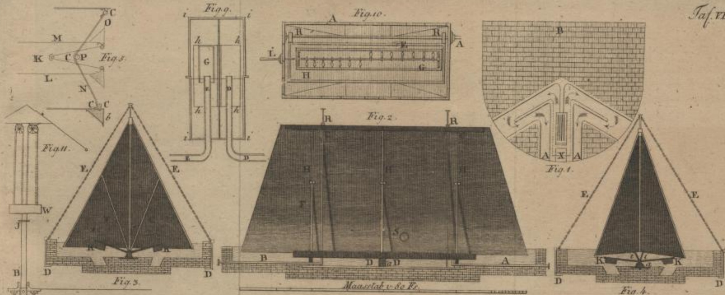
Gas-Behälter zu Chester von 50,000 Cubic Fc. Gehalt.
