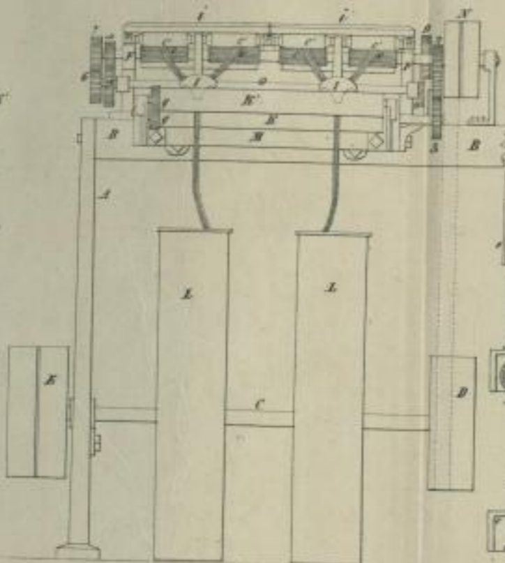
Streckwerk. Vorderer Ansicht der einen Walzenreihe.
