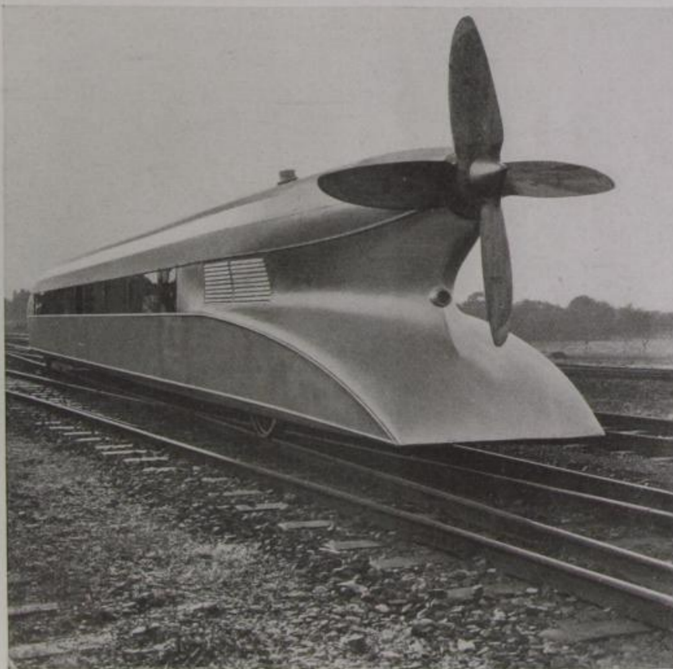
Der neue Schienenzeppelin
