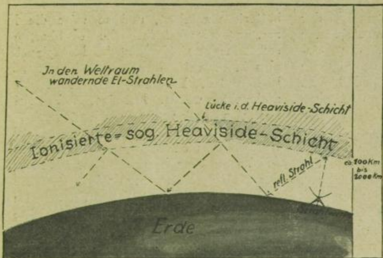
Veranschaulichung der neuesten Hypothese über das Wandern der El-Wellen in den Weltraum durch die ionisierte Schicht hindurch
