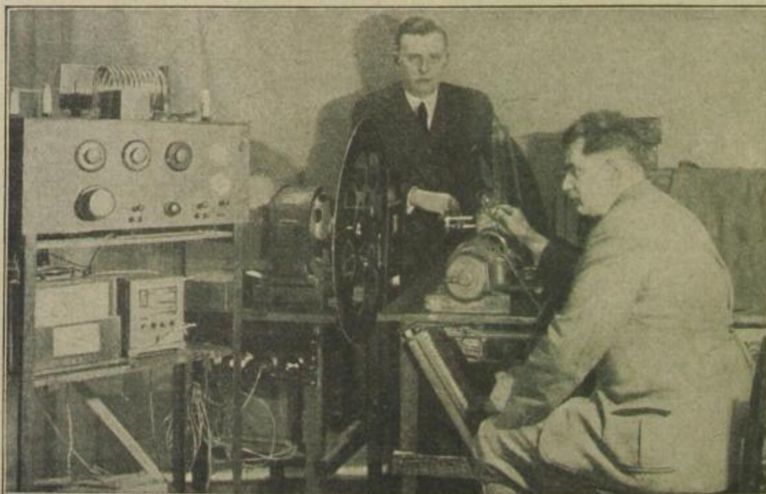
Sendeanlage für Kino-übertragung mit Funk-sender. Dahinter, ste-hend: Der Erfinder Denes v. Mihaly Copyright by Telehor Akt.-Ges.
