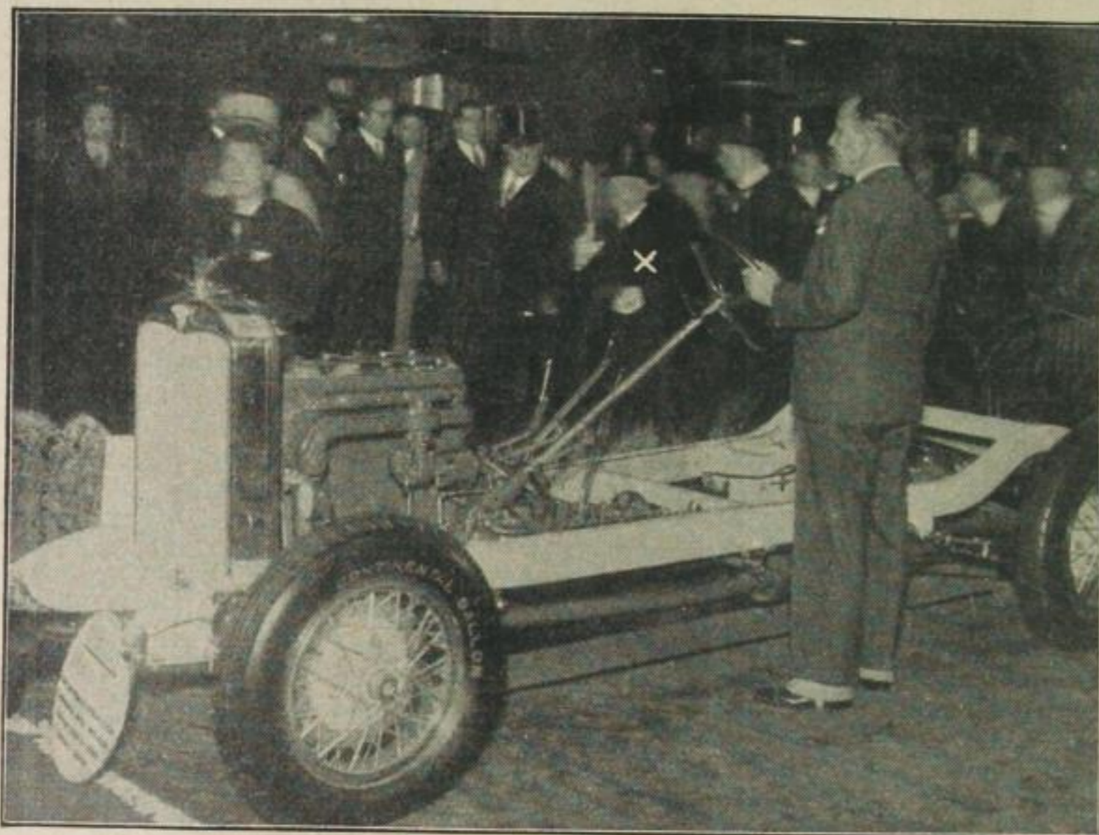
Auf der Ausstellung der Firma Wanderer-Werke, Schönau, im Pariser-Automobil-Salon fiel das neue hervorragend durchkonstruierte Chassis des 10/50 P. S. Sechs-Zylinder-Wagens besonders auf. Das Bild zeigt die Besichtigung durch den Präsidenten der französischen Republik (x)
