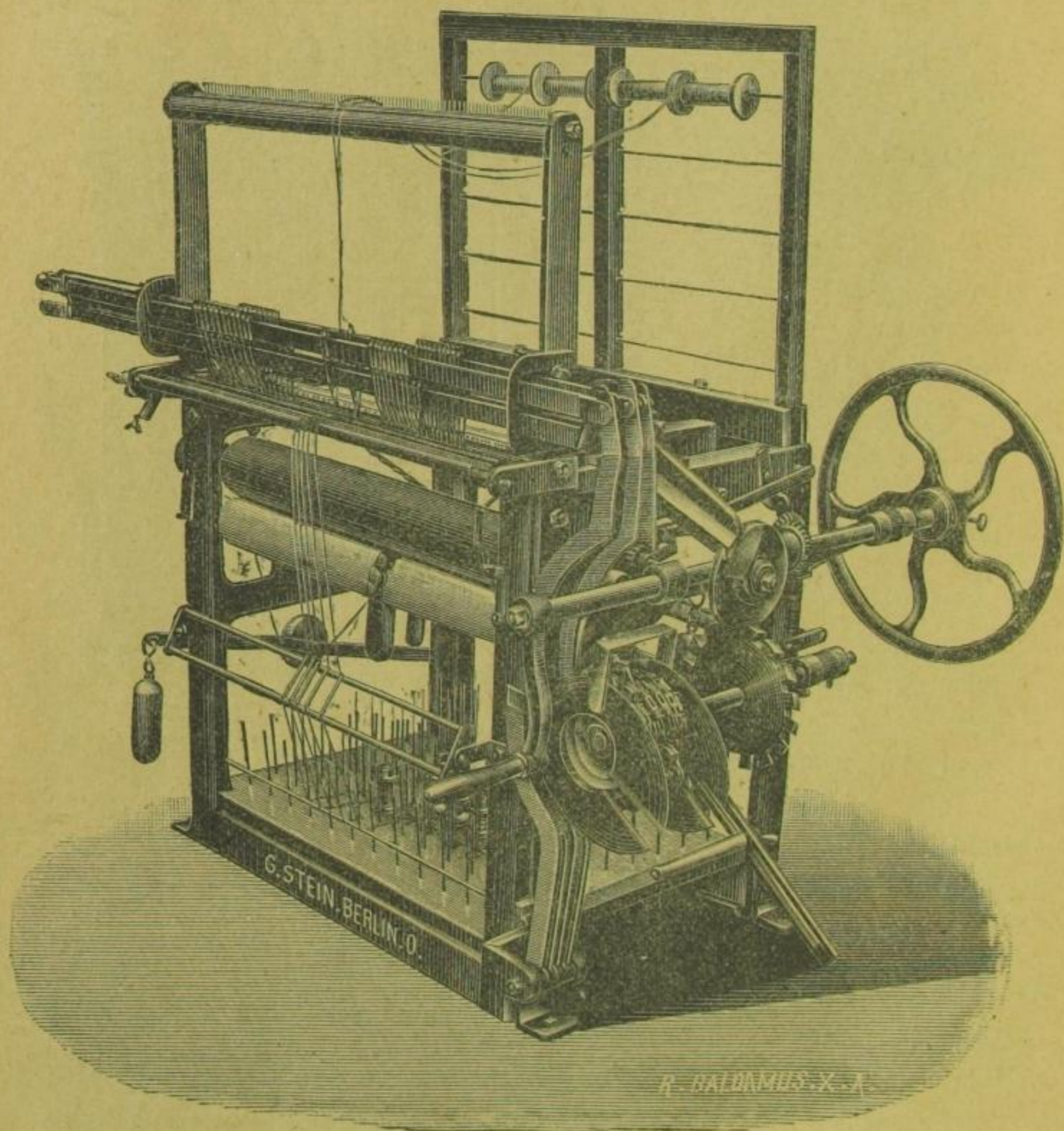
Galon-Kästelmaschine.
