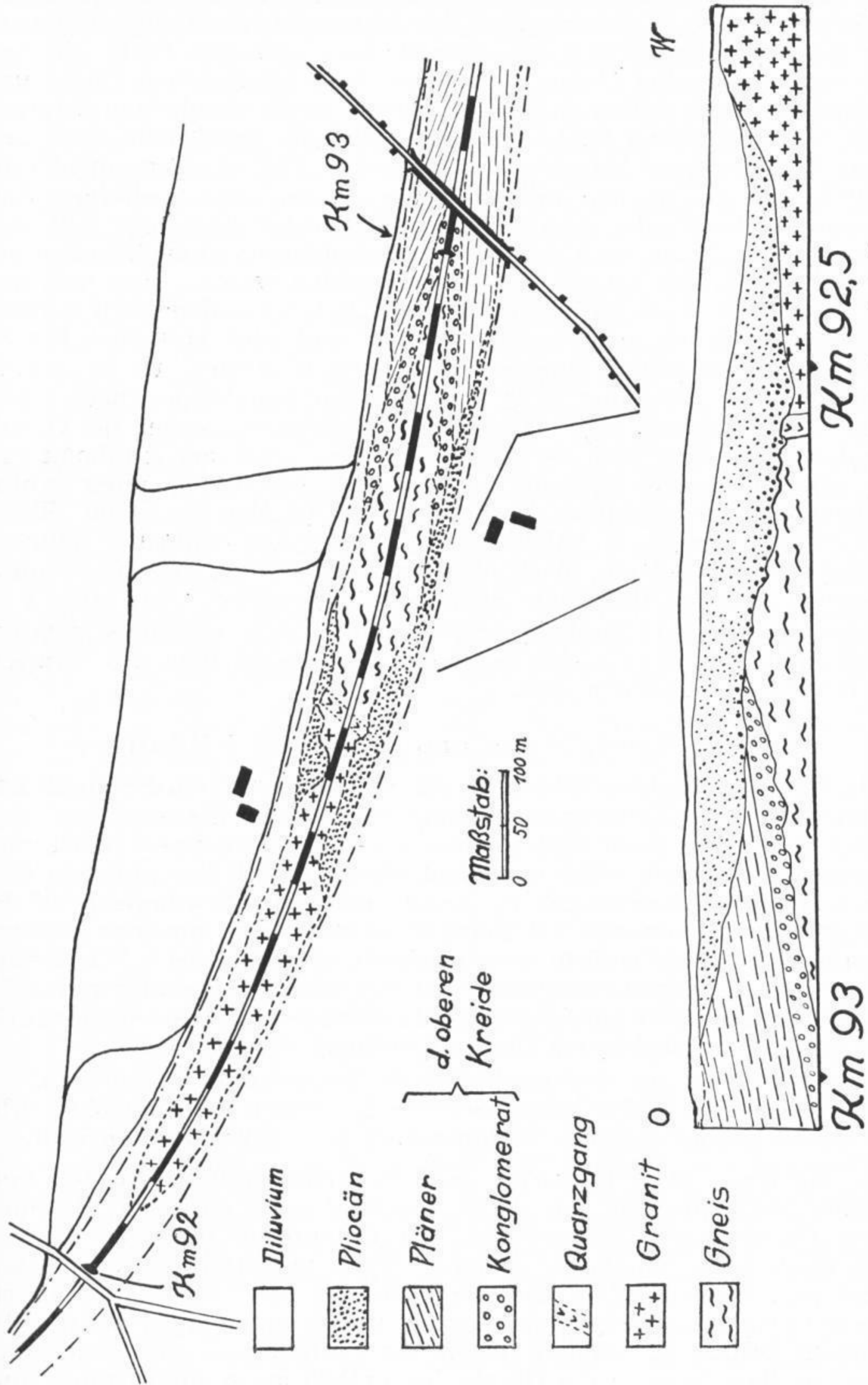
Abb. 2: Geologische Karte und Profil (6× überhöht) des Eisenbahneinschnittes bei Oberau (nach Aufnahmen von H. HÖPPNER und eigenen Beobachtungen)
