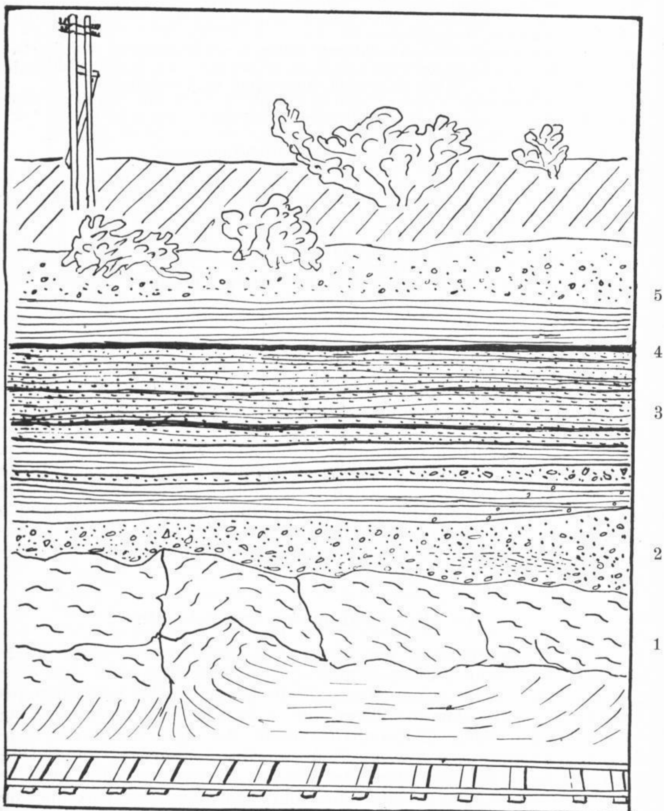
Abb. 3. Teilprofil des Pliocäns am Südhang des Anschnittes von Oberau (Zeichnung nach einer photographischen Aufnahme des Verfassers).
