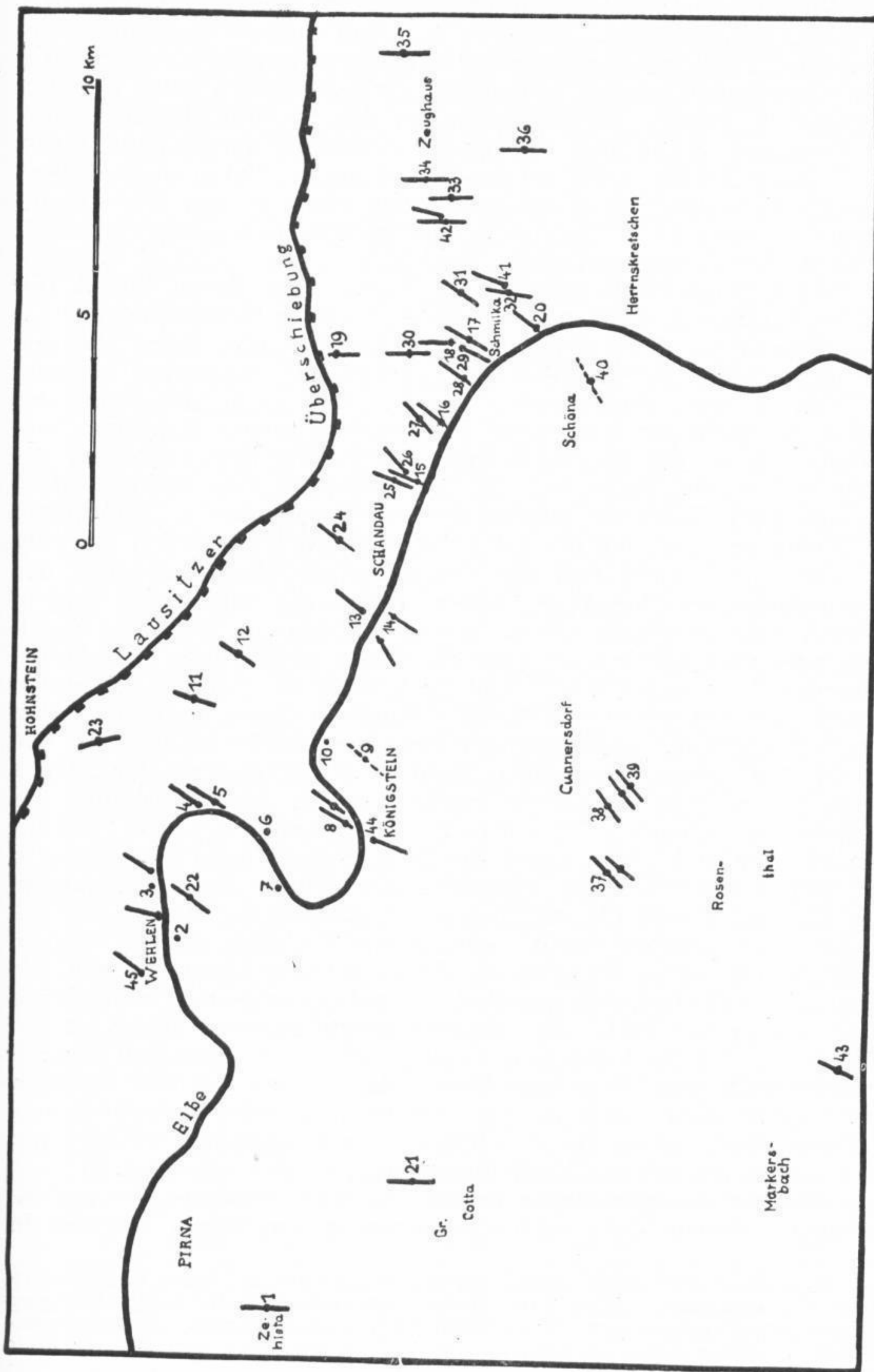
Abb. 2: Verbreitung und Richtung der bisher bekannten Vorkommen von Wellenfurchen im Elbsandsteingeirge
