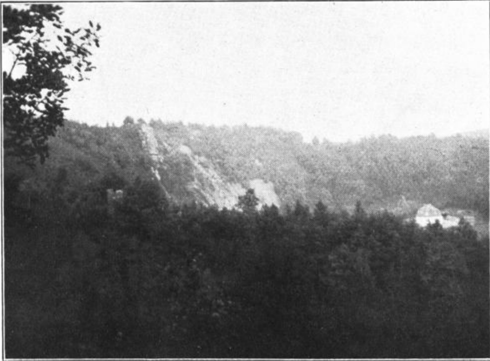
Abb. 1: Der Quarzit östlich des Baratales.
