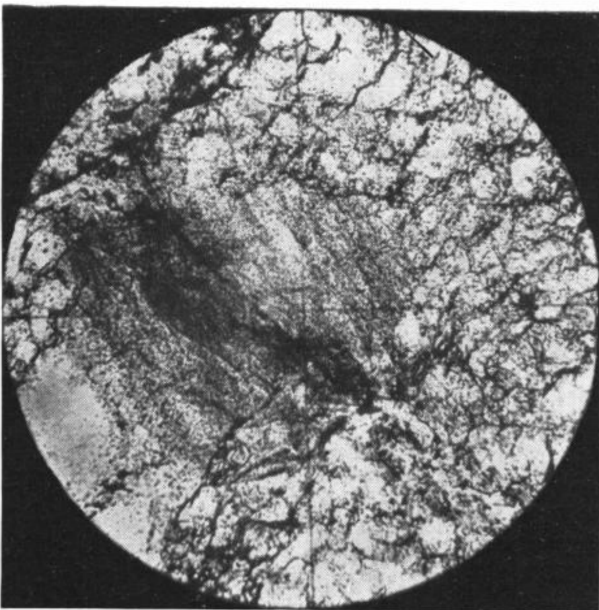
Abb. 3: Beginnende Zertrümmerung eines Quarzkornes. 20 × Vergr.
