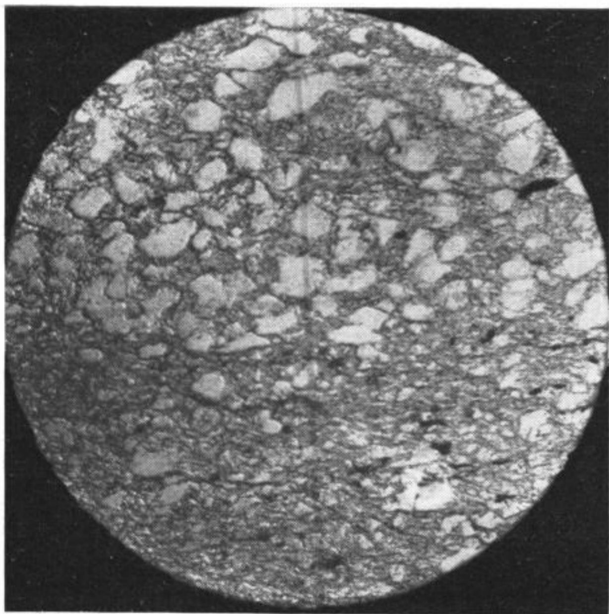
Abb. 1: Quarzit mit gerundeten Körnern. 12 × Vergr.
