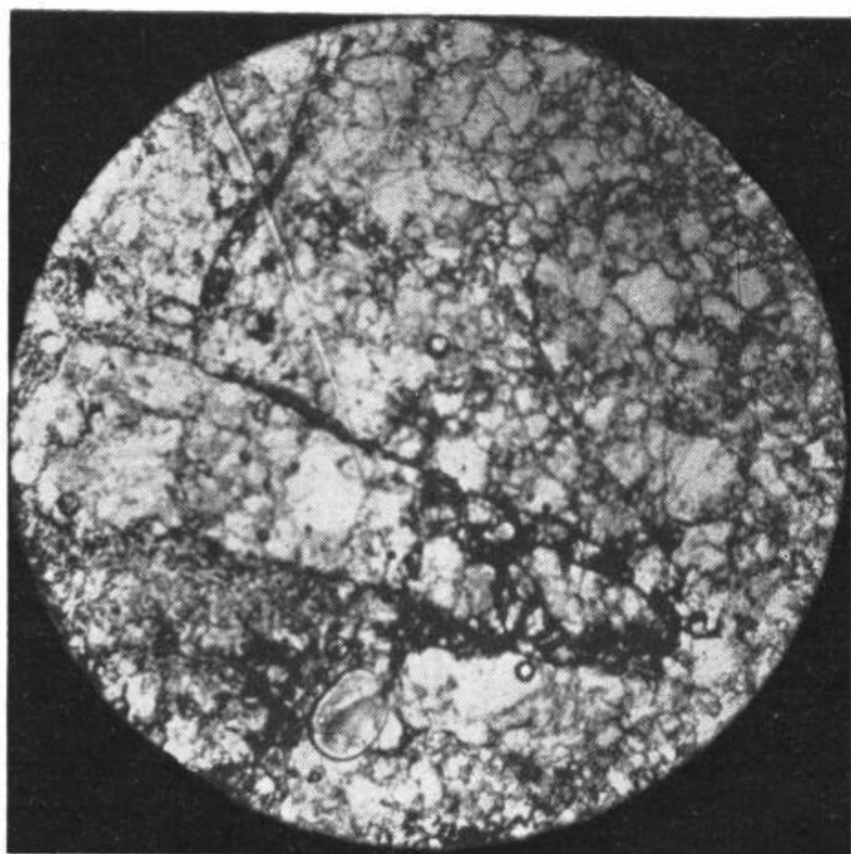
Abb. 4: Brecciöser Quarzit. 13 × Vergr.
