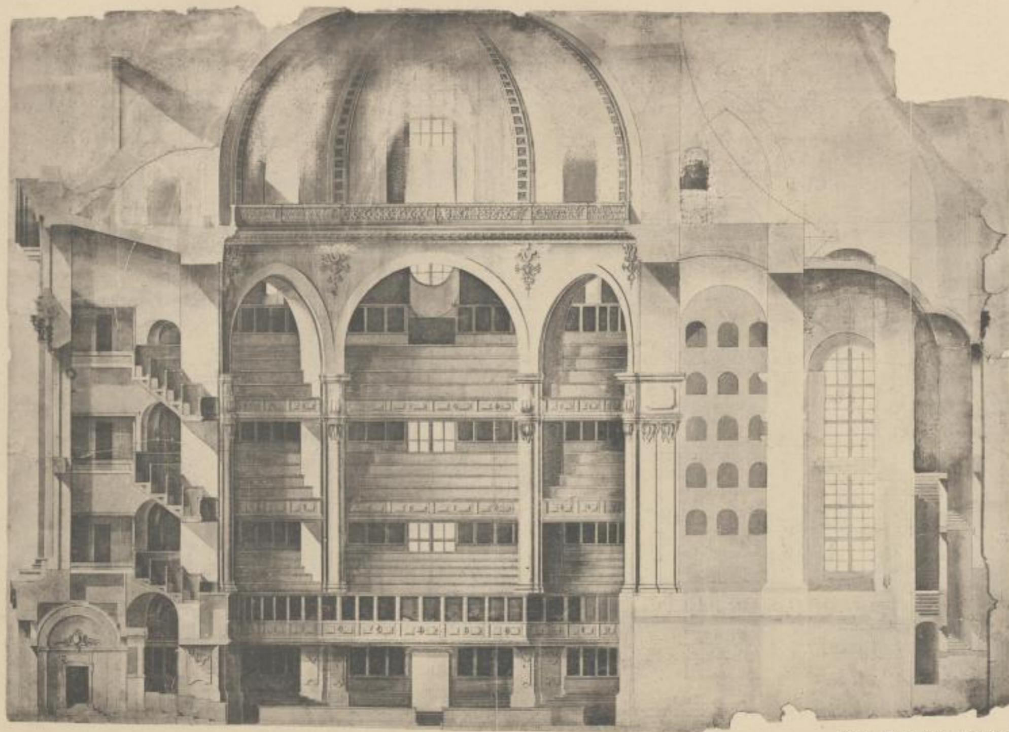
Längenschnitt des dritten Projekts mit Steinkuppel.
