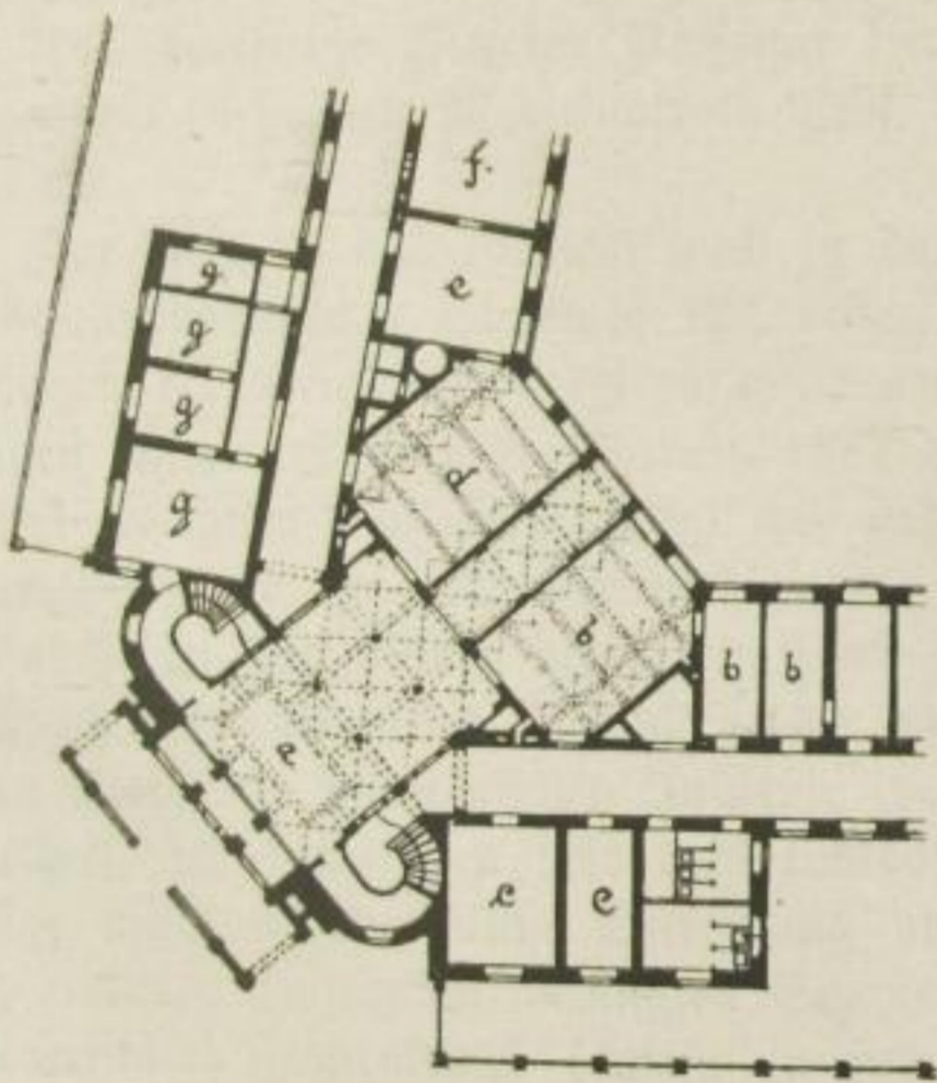
Unteres Erdgeschoss.
