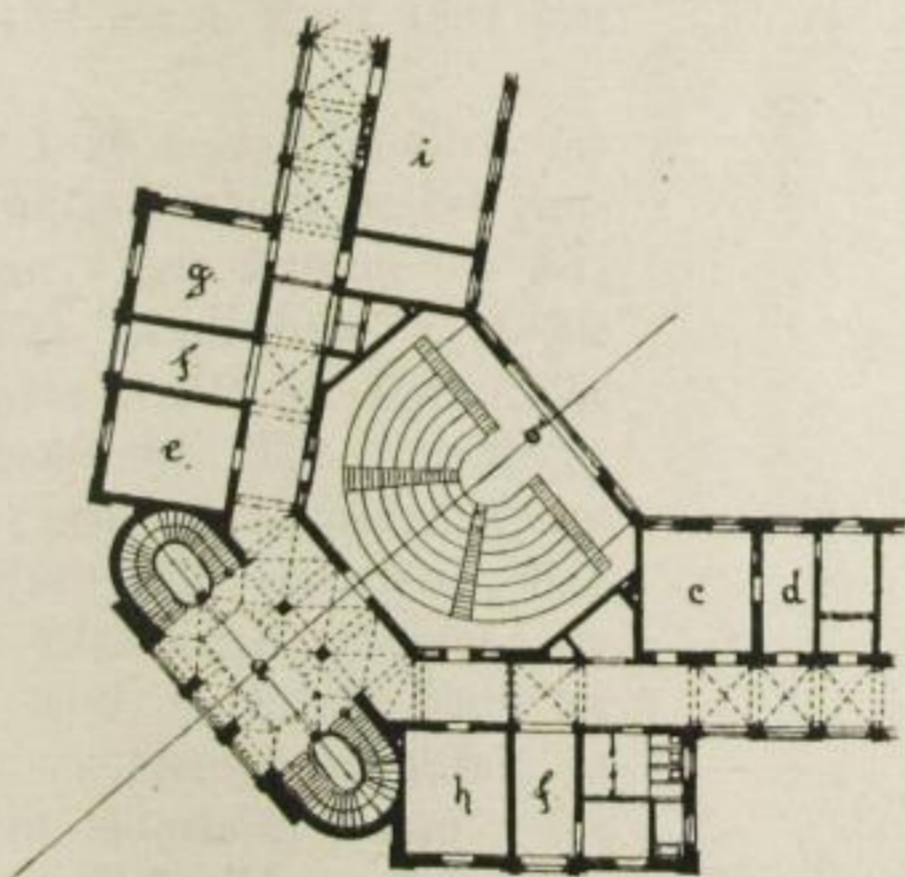
2. Obergeschoss.
