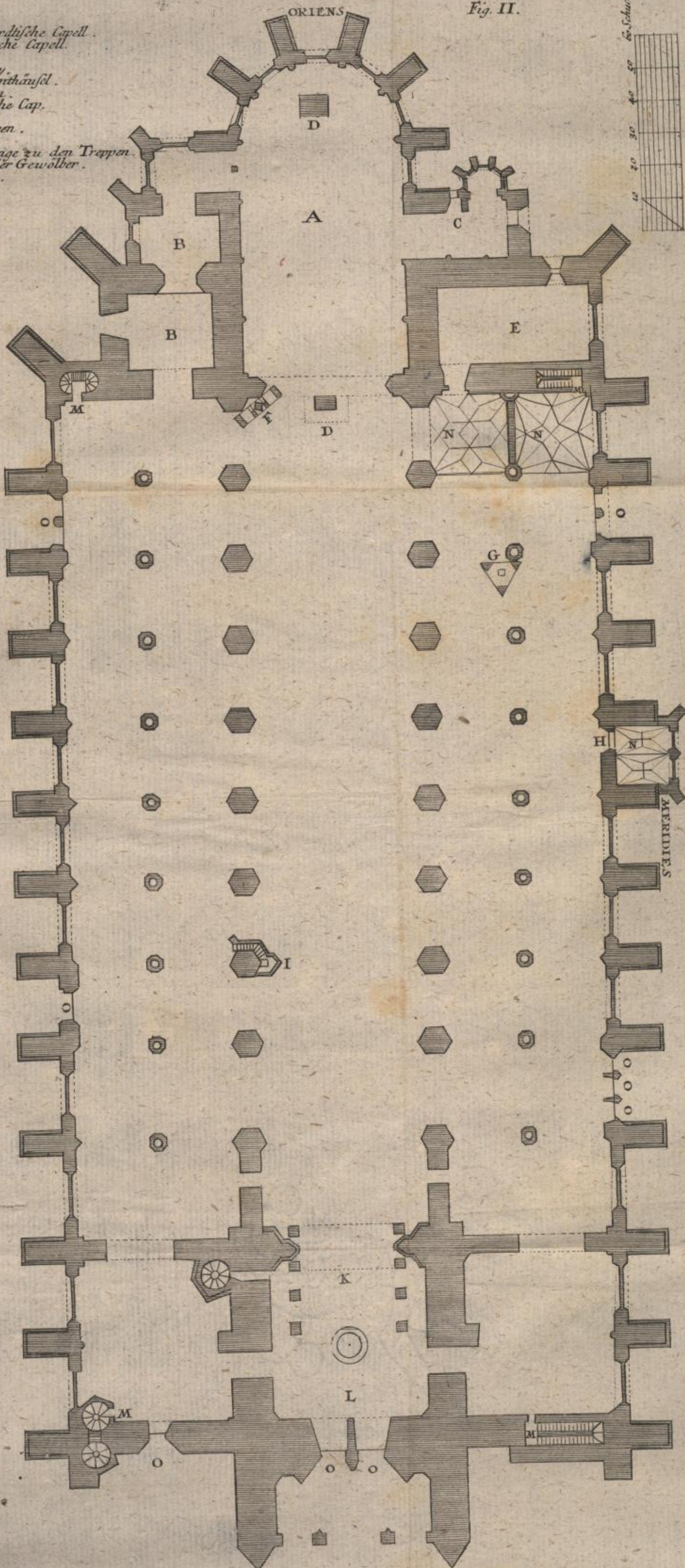
Grundriß des Münsters zu ULM.
