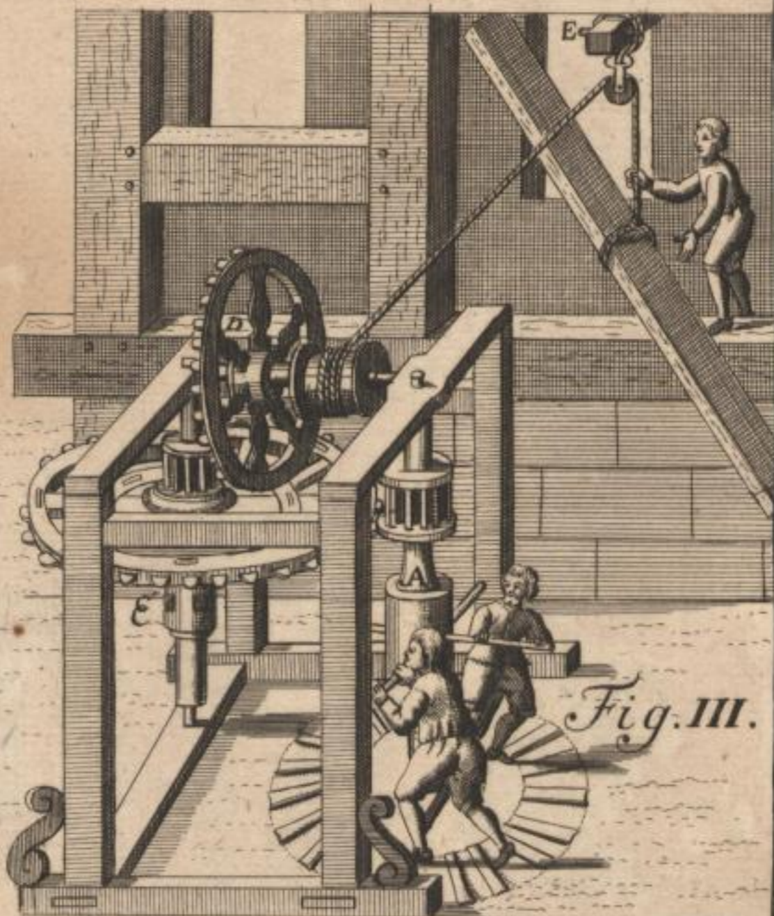
Fig. III. A. Getriebe mit dem Haspel B. Stirn-Rad mit dem Getriebe D. Kam-Rad.
