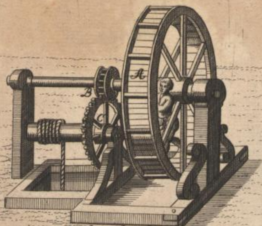
Fig. IV. A. Trot-Rad B. Getriebe C. Stirn-Rad.
