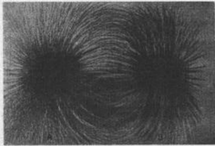
Abb. 3 Feilspanbild in der Draufsicht der Pole. A = Kraftlinienfluß des Hohlmagneten gleichmäßig an der ganzen Polfläche, B = do. Vollmagnet nur an den Rändern der Polfläche
