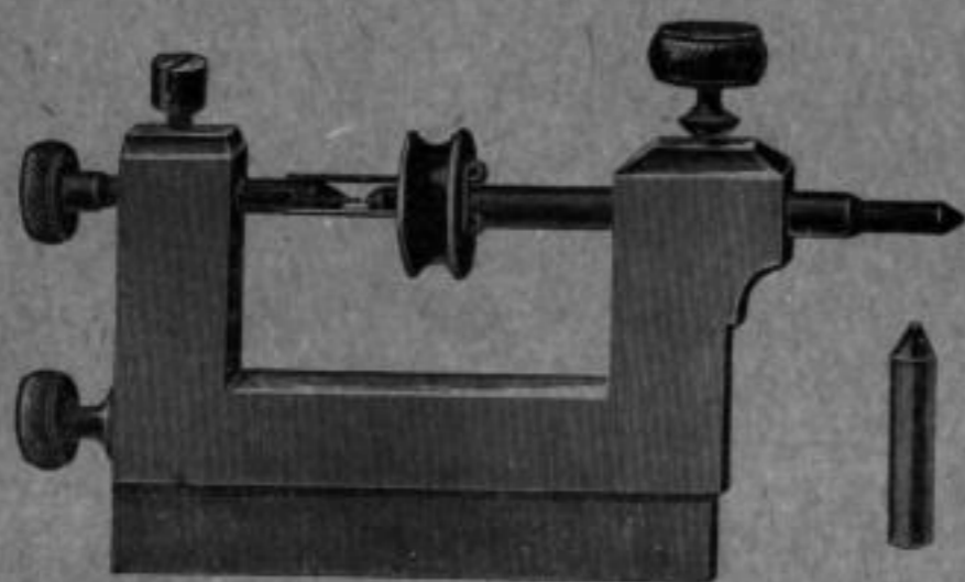
Nr. 1959. Zapfenbohrmaschinen
