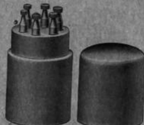
Nr. 6094. Fassungsräser
