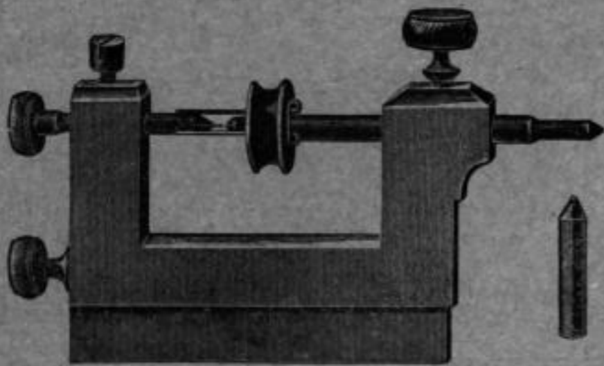
Nr. 1959. Zapfenbohrmaschinen
