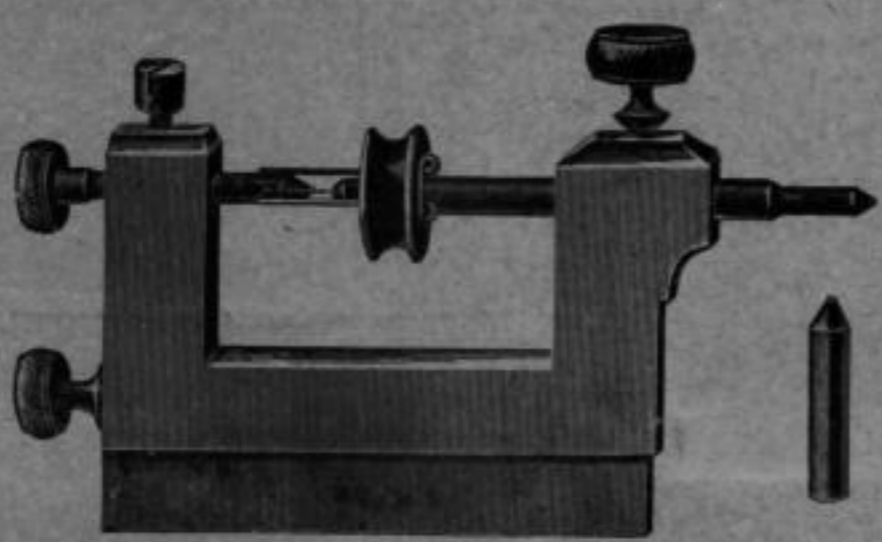
Nr. 1959. Zapfenbohrmaschinen
