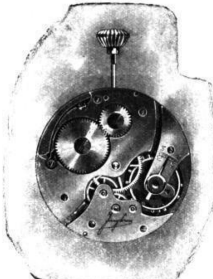
Abb. 19. Meisterwerk J 13 (offen)
