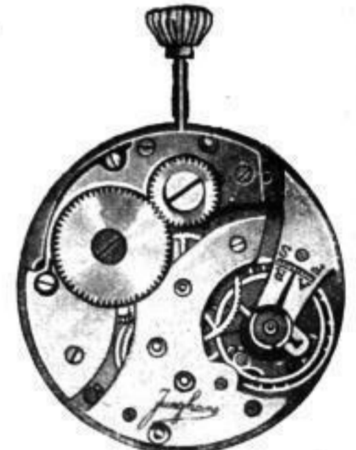
Abb. 17. Werk der Uhr J. 9
