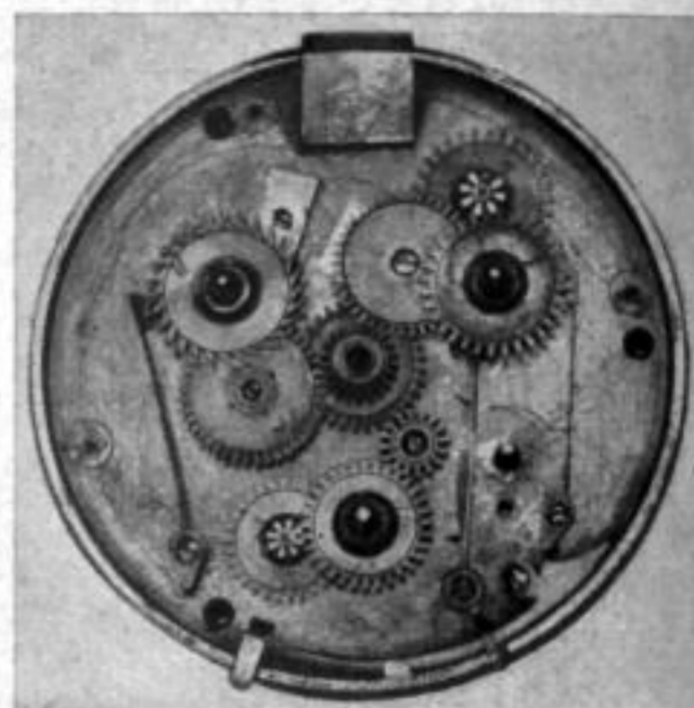
Abb. 29 Kalender-Taschenuhrwerk, frühe Arbeit der Brüder Georg und Christian Hahn; das Zifferblatt noch auf Echterdingen lautend, mit Spruch: „Elles sont toutes marquées.“ Besitzer: Ferd. T. Haschka, New York
