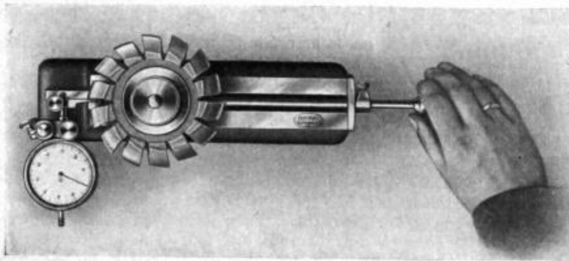
Prüfen des richtigen Anschliffs der Schneidbrust der Fräserzähne
