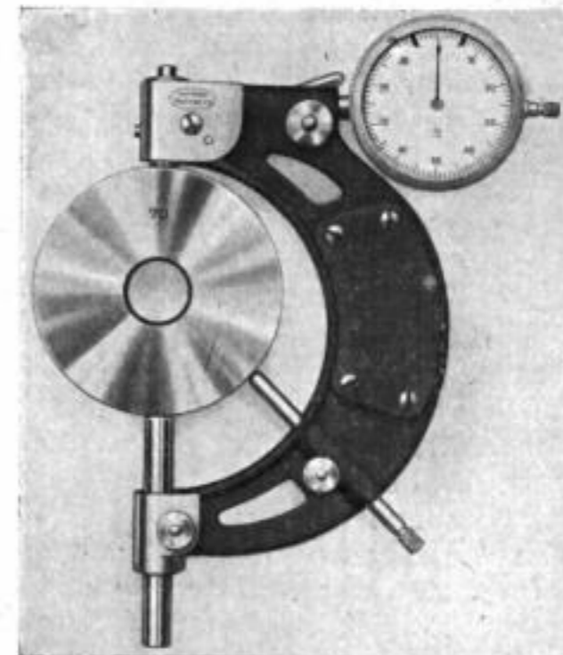
Rachenlehre mit Meßuhr
