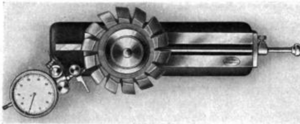
Prüfung eines Fräsers auf Rundlauf
