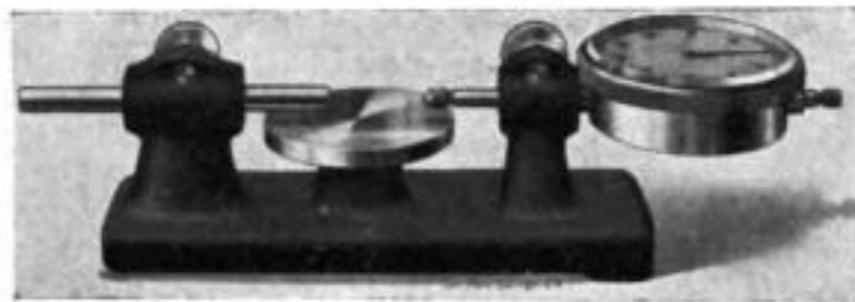
Meßfisch mit wagrechter Anordnung der Meßuhr
